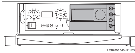
Fig. 3 Betjeningsenhed (eksempel ModuLine 400)
