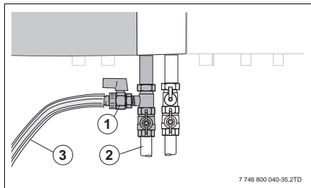
Fig. 10 Åbning af påfyldnings- og aftapningshanen
