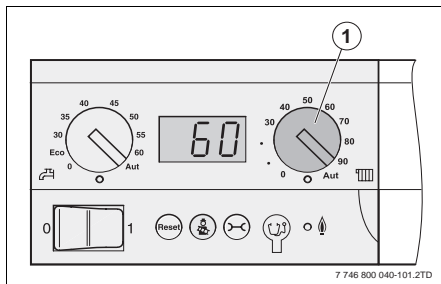
Fig. 6 Basiscontrollers betjeningspanel
