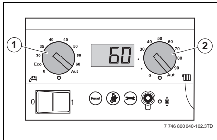
Fig. 8 Betjeningspanel basiscontroller
