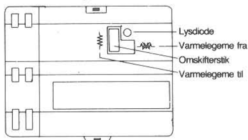
Varmelegeme-relæ
