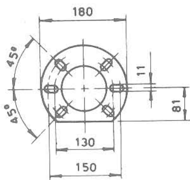
Flange
