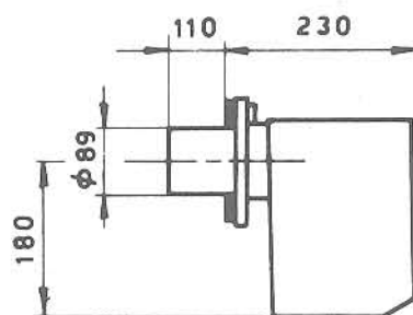
Oliefyret
