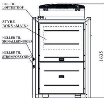
Forfra
