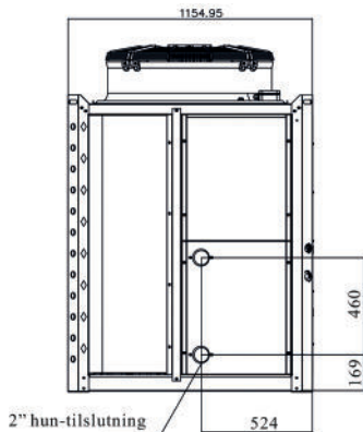
Fra siden
